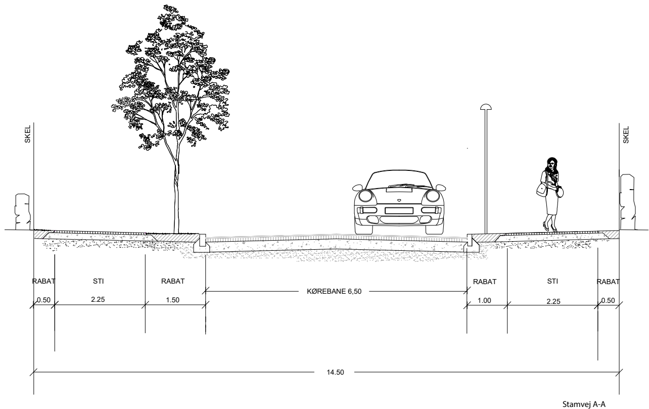
Figur 10: Snit af stamvejens udformning.
